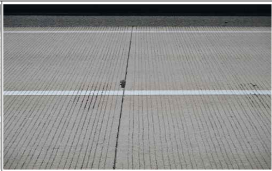
교면포장 하행선 S1 포장면 박락
