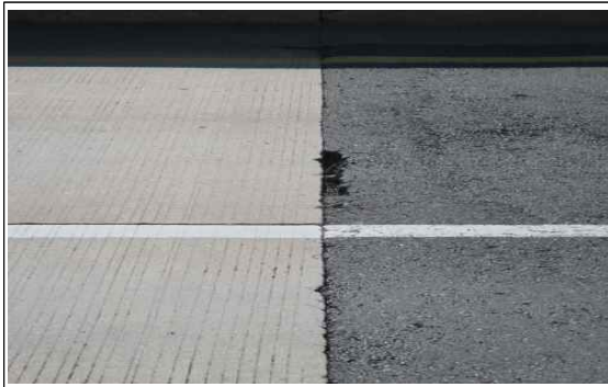
교면포장 상행선 A1측 접속도로 패임
