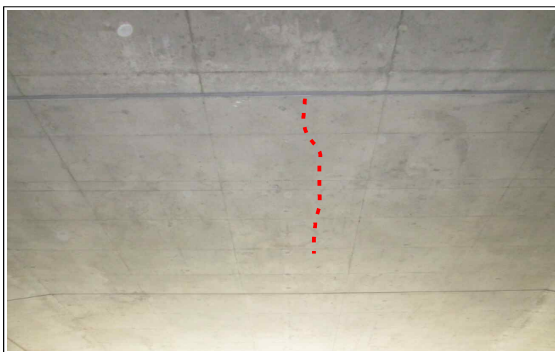
바닥판하면 상행선 S1 균열(폭 0.1mm)
